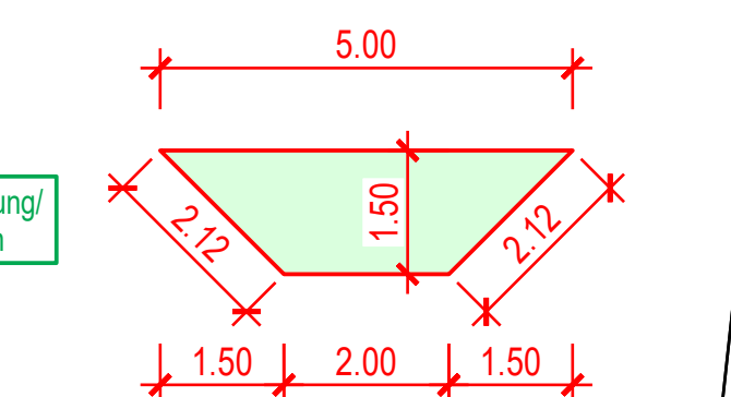
Detail Verkehrsberuhigung 1:100
